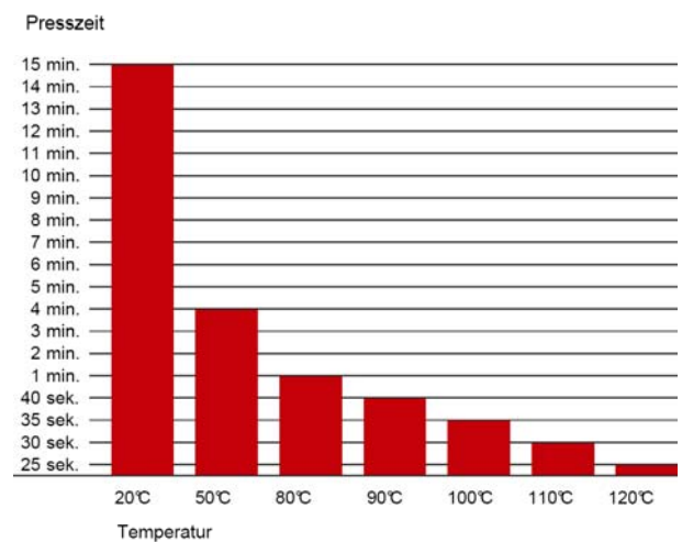
Presszeiten für 0,6 mm Buchenfurnier auf Spanplatte
